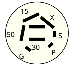
Zündanlassschalter Schema
