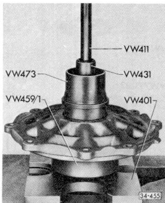
Abb. 6 Außenring/Kegelrollenlager für Ausgleichgetriebe auspressen
