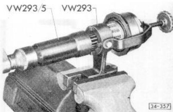
Abb. 6 Rundmutter in Vorrichtung VW 293 lösen bzw. anziehen.
