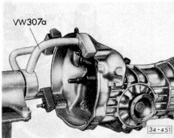
Abb. 1 Getriebe in den Montagebock spannen AUDI NSU: Halter VW 540.
