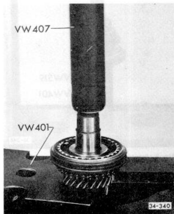
Abb. 2 Schiebemuffe/Synchronkörper mit Zahnrad für 3. Gang abpressen
