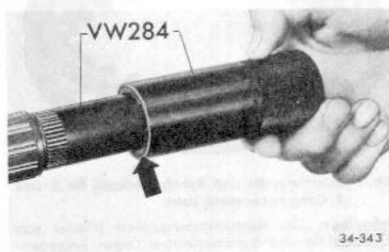
Abb. 5 Sicherungsring aufsetzen
