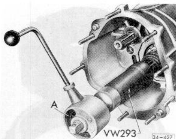
Abb. 15 Reibmoment des Doppelkegelrollenlagers prüfen
