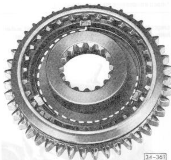
Abb. 11 Federn einsetzen
