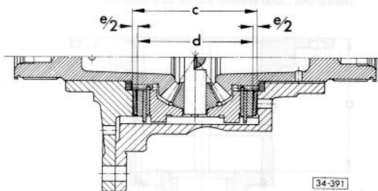
Abb. 7 Maß „e“ ermitteln
