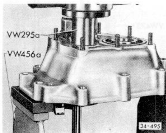
Abb. 8 Nadellager für Triebling einpressen
