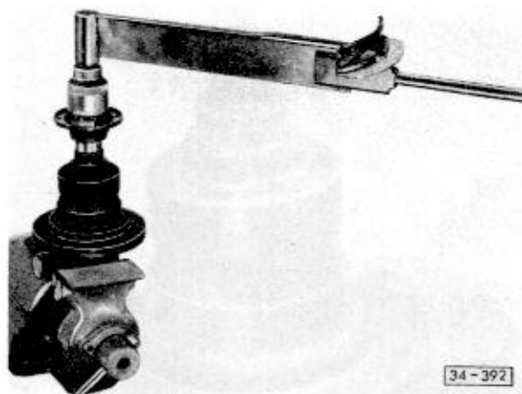
Abb. 8 Nach dem Zusammenbau Drehmoment prüfen
