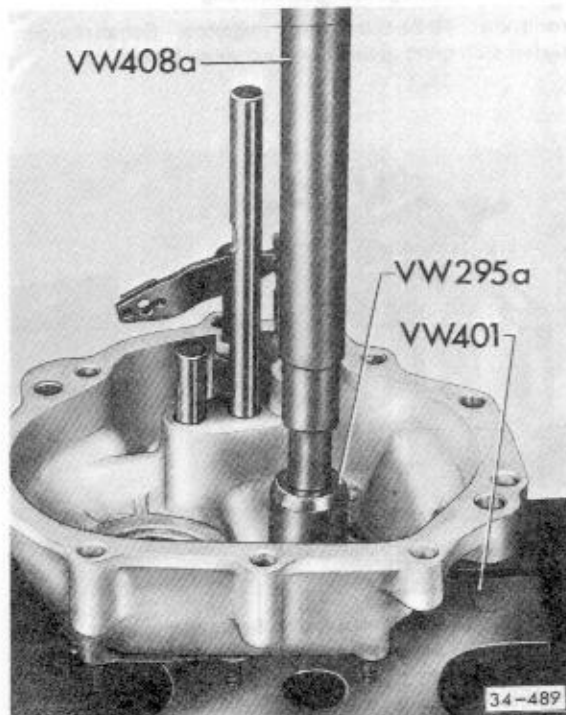
Abb. 2 Nadellager für Triebbling auspressen AUDI NSU: Einsteckdorn 30-505 und Druckteller 30-206.
