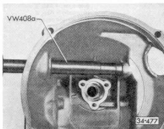
Abb. 8 Lagerbuchse für Ausrückwelle bündig eintreiben
