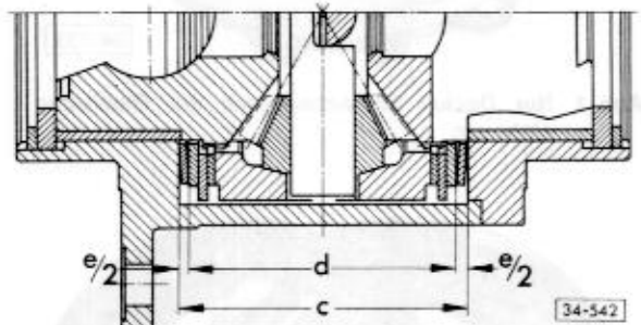
Abb. 8 Maß „e“ ermitteln
