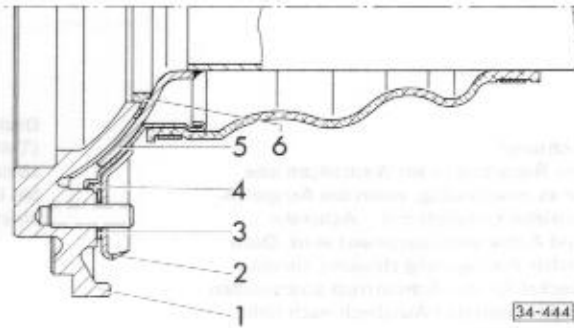
Abb. 14 Achsrohr einstellen
