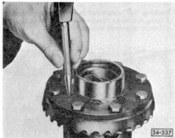
Abb. 11 Innensechskantschrauben mit 25 Nm (2,5 mkg) anziehen und durch Körnerschlag sichern
