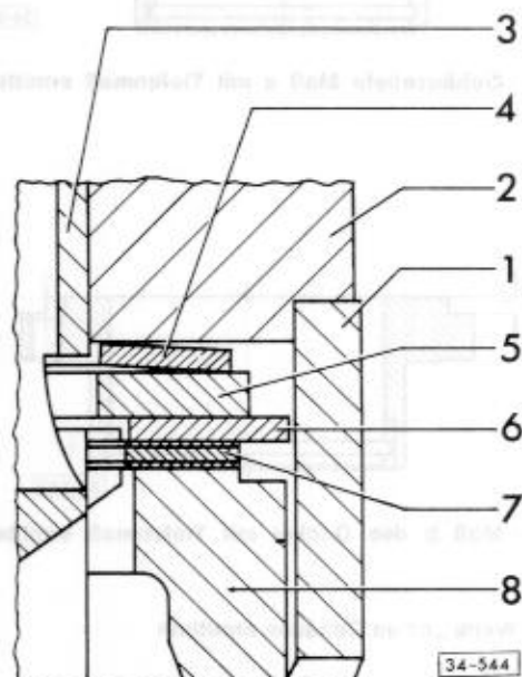
Abb. 4 Einbaulage der Lamellen
