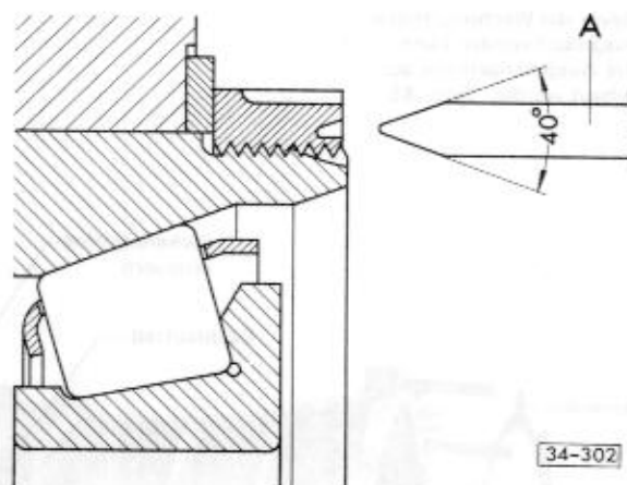
Abb. 4 Spannmutter durch Verstemmen sichern A – Selbstgefertigtes Stemmwerkzeug.
