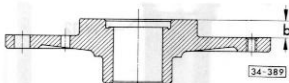
Abb. 5 Maß b des Deckels mit Tiefenmaß ermitteln
