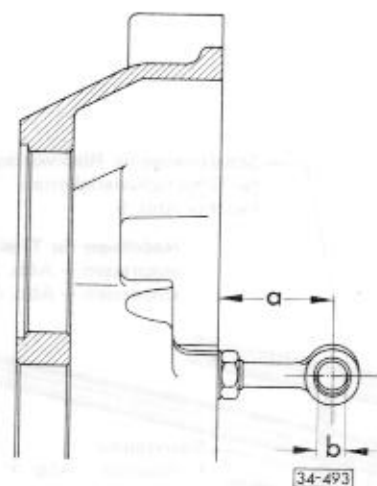
Abb. 6 Stütze für Umkehrhebel einstellen
