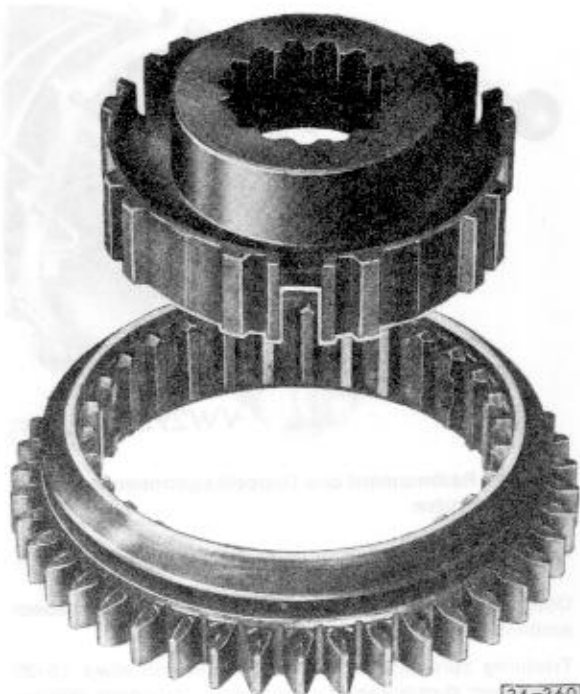
Abb. 10 Schiebemuffe und Synchronkörper für 1. und 2. Gang zusammenbauen
