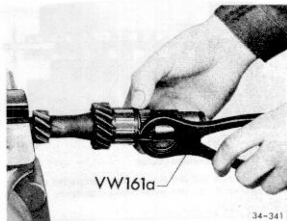
Abb. 3 Sicherungsring abnehmen
