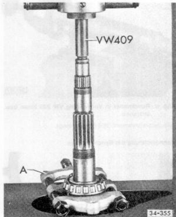
Abb. 4 Innenring abpressen
