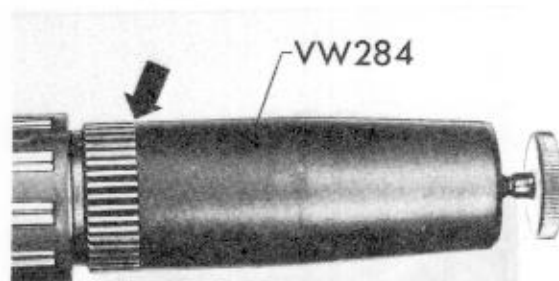
Abb. 4 Sicherungsring aufsetzen
