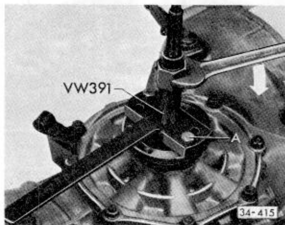
Abb. 3 Gelenkflansch abziehen
