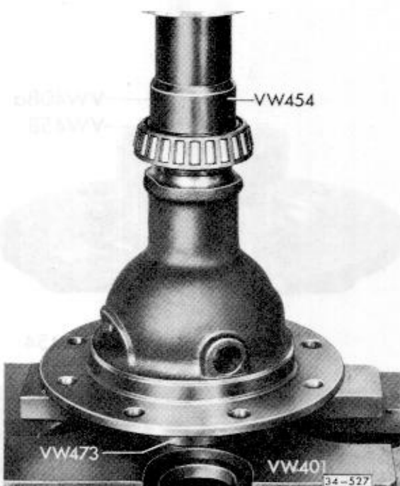
Abb. 6 Innenring/Kegelrollenlager auf ca. 100° C erwärmen, aufsetzen und nachpressen
