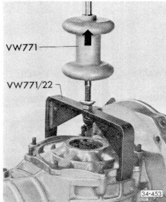
Abb. 4 Deckel für Achsantrieb abziehen
