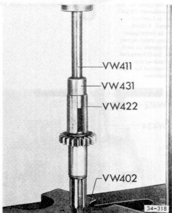
Abb. 11 Sicherungsring in die Nut pressen
