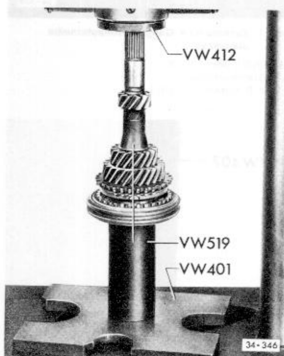
Abb. 9 Schiebemuffe mit Synchronkörper aufpressen
