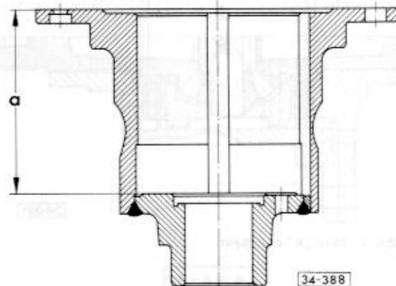
Abb. 4 Gehäusetiefe Maß a mit Tiefenmaß ermitteln
