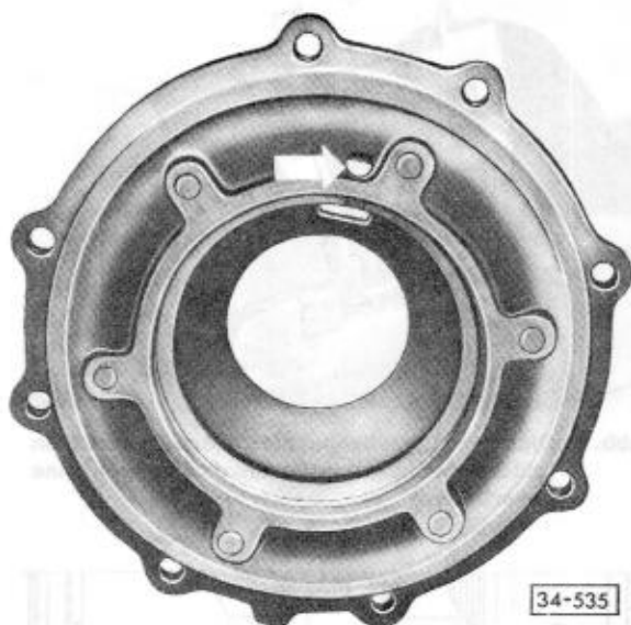
Abb. 1 Nur Deckel für Achsantrieb mit Ölbohrung einbauen
