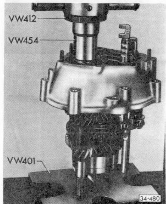
Abb. 2 Antriebswelle mit Triebbling einpressen AUDI NSU: Einpreßwerkzeug 41-501.
