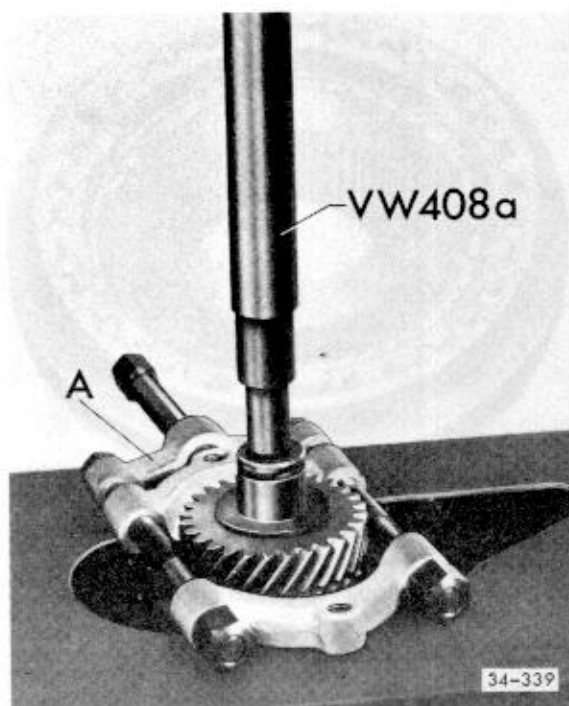
Abb. 1 Zahnrad für 4. Gang und Anlaufscheibe abpressen
