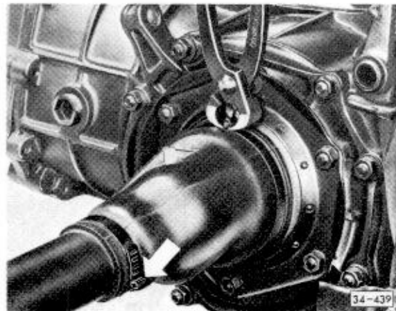
Abb. 9 Schlauchbinder mit Klemmzange (handelsüblich) zuziehen
