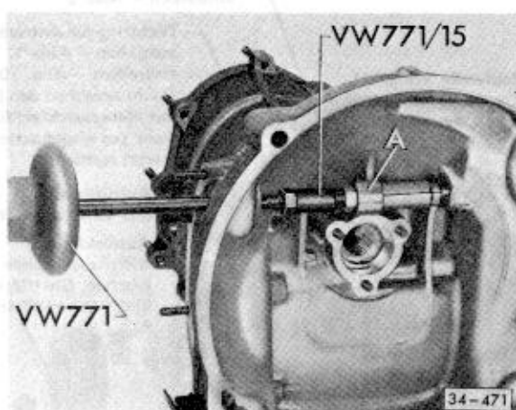
Abb. 2 Lagerbuchse für Ausrückwelle ausziehen
