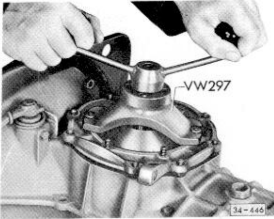
Abb. 1 Deckel für Achsantrieb abziehen
