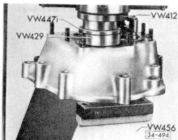
Abb. 7 Rillenkugellager für Antriebswelle einpressen
