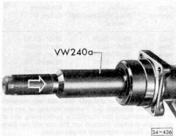
Abb. 6 Rillenkugellager eintreiben
