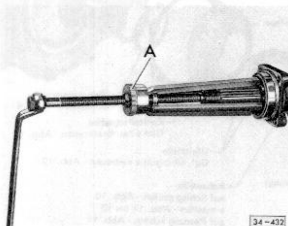
Abb. 2 Rillenkugellager abziehen A – Innenauszieher z. B. Kukko 70/2 mit Haken 722
