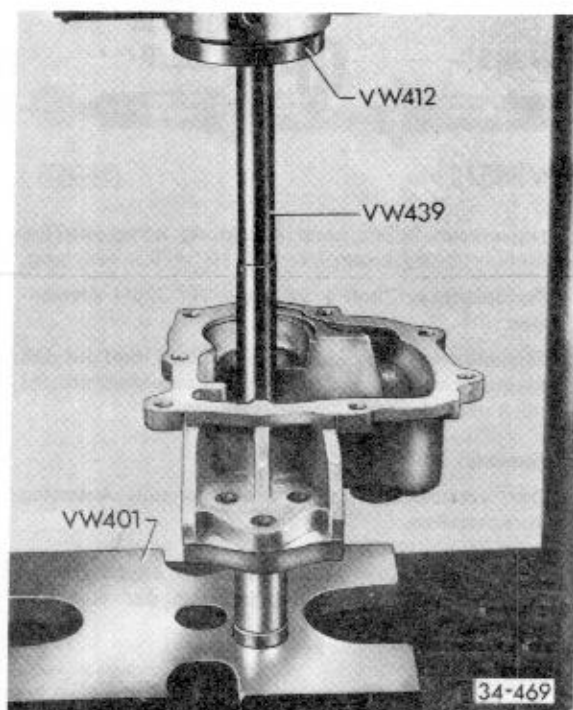
Abb. 3 Lagerbuchse innen, bündig einpressen
