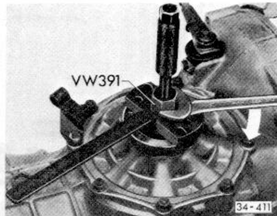
Abb. 12 Gelenkflansch aufziehen
