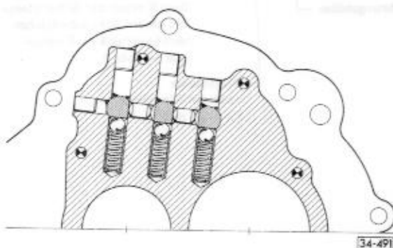
Abb. 4 Einbaulage Gangarretierung
