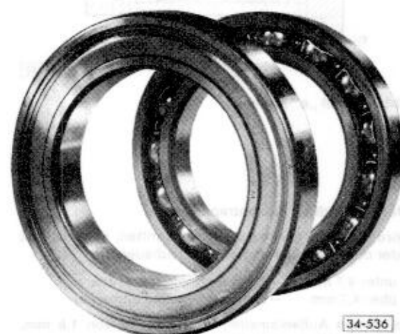
Abb. 2 Rillenkugellager so einbauen, daß die geschlossene Seite des Käfigs im Deckel für den Achsantrieb liegt
