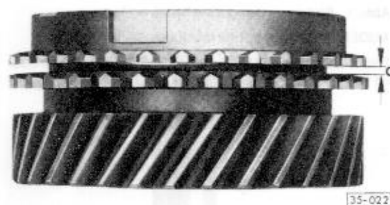
Abb. 8 Synchronringe prüfen
