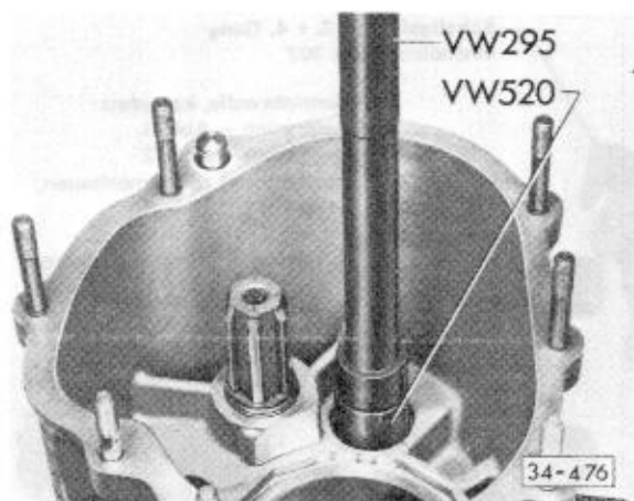
Abb. 7 Nadellager für Antriebswelle eintreiben
