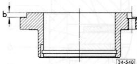
Abb. 6 Maß b des Deckel mit Tiefenmaß ermitteln
