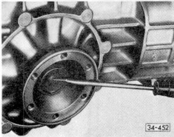
Abb. 2 Verschlusskappe heraushebeln
