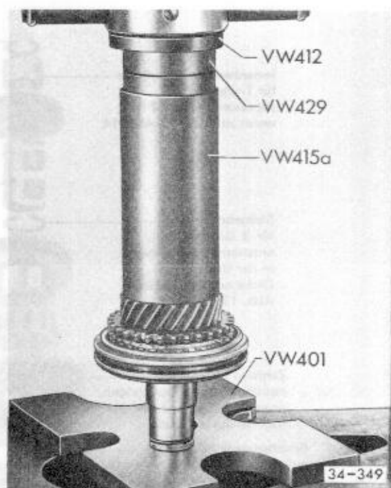
Abb. 12 Synchronkörper zurückdrücken
