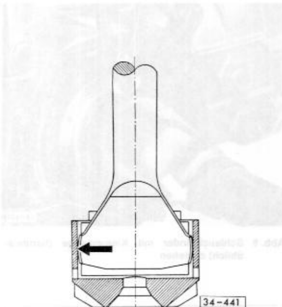
Abb. 11 Achswelle einstellen
