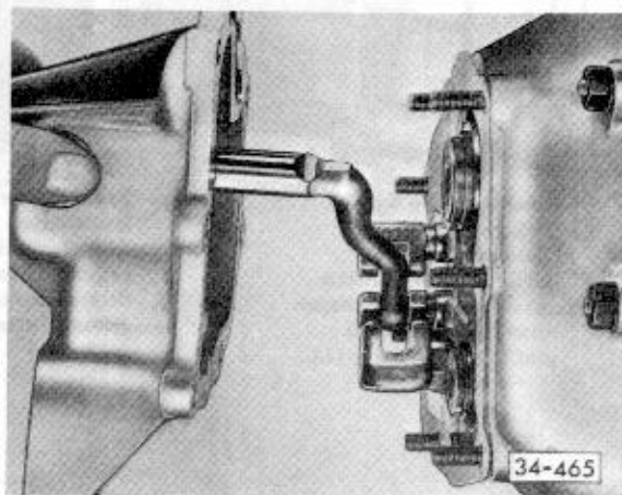
Abb. 5 Innenschalthebel in die Schaltstangen einsetzen
