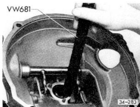
Abb. 1 Dichting für Antriebswelle ausziehen
