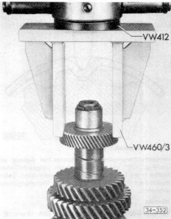
Abb. 1 Sicherungsring abnehmen
