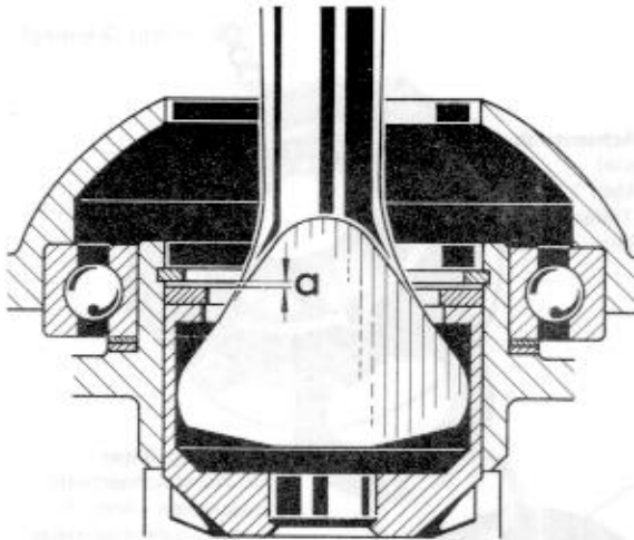
Abb. 13 Achswelle einstellen
