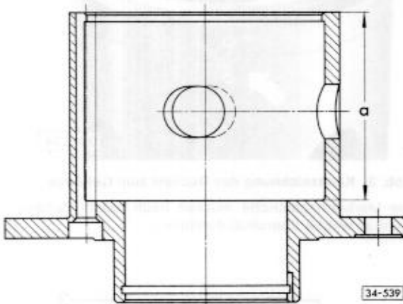
Abb. 5 Gehäusetiefe Maß a mit Tiefenmaß ermitteln
