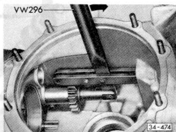
Abb. 5 Komplette Rücklaufwelle eindrücken. Dazu gegebenenfalls Ausdrückhebel nach Abb. 6 umarbeiten.
