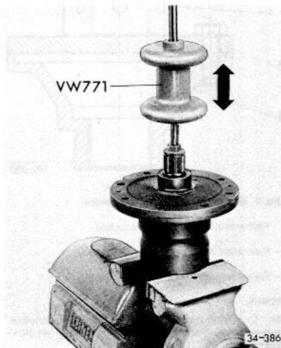
Abb. 2 Deckel vom Gehäuse abziehen
