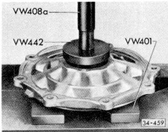
Abb. 10 Dichtring einpressen
