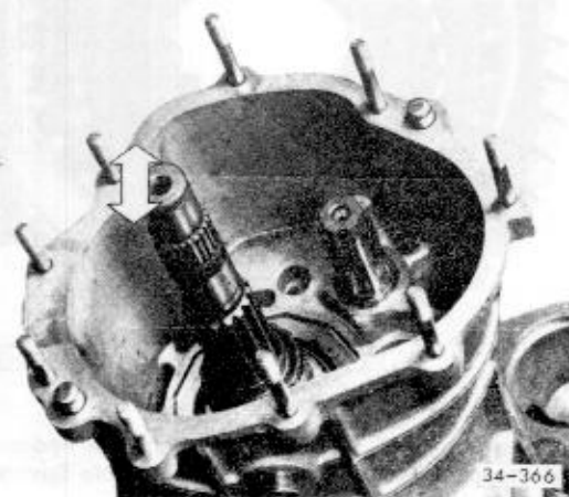
Abb. 16 Kippspiel/Doppelkegelrollenlager prüfen.
