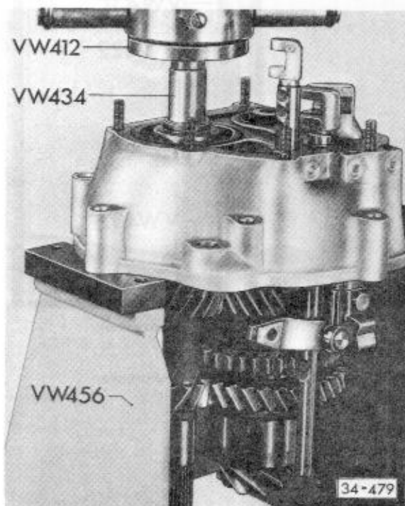
Abb. 1 Antriebswelle mit Triebbling auspressen AUDI NSU: Hülse 12-550 und VW 456 a.
