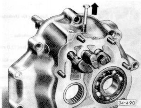
Abb. 3 Verschlussstopfen ausziehen
