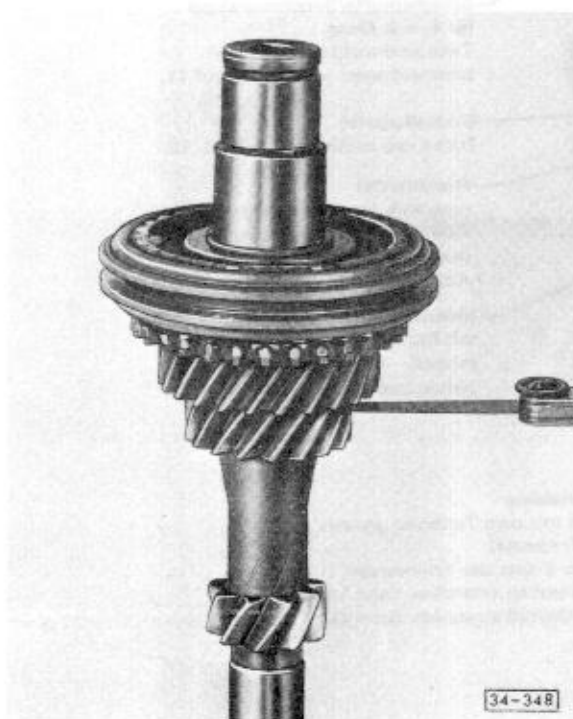
Abb. 11 Spiel zwischen 2. + 3. Gangrad mit einer Fühlerblattlehre messen
