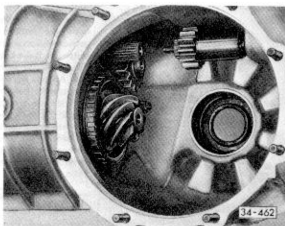
Abb. 1 Vordere und hintere Antriebswelle auseinander-schrauben
