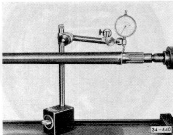
Abb. 10 Achswelle auf Schlag prüfen. Zulässig: 0,05 mm
