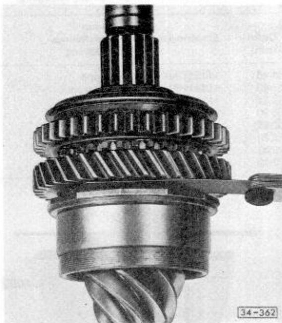
Abb. 12 Axialspiel des Zahnrades für 1. Gang einstellen
