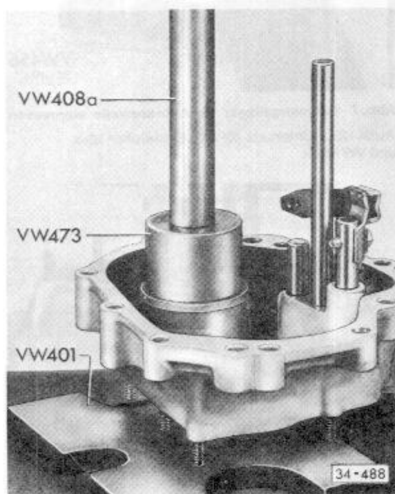
Abb. 1 Rillenkugellager für Antriebswelle auspressen AUDI NSU: Einsteckdorn 30-505 und Aufpreßstück 40-202.
