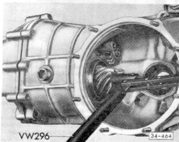
Abb. 3 Wechselgetriebe herausdrücken
