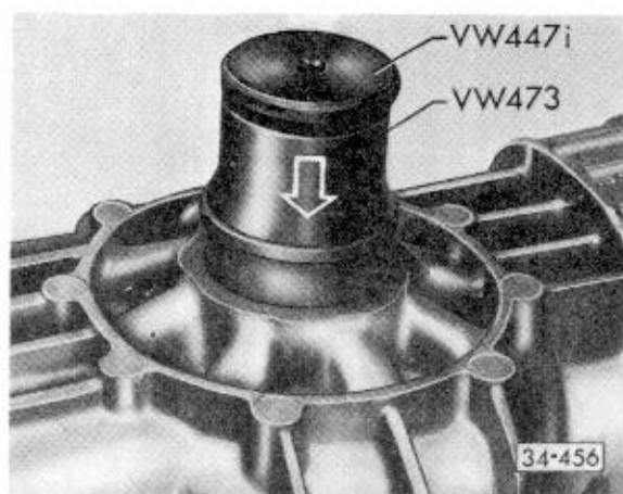
Abb. 7 Außenring/Kegelrollenlager für Ausgleichgetriebe mit Plastikhammer austreiben
