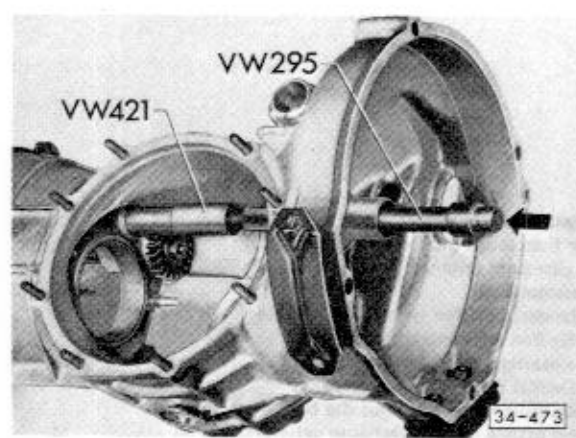
Abb. 4 Nadellager für Antriebswelle austreiben
