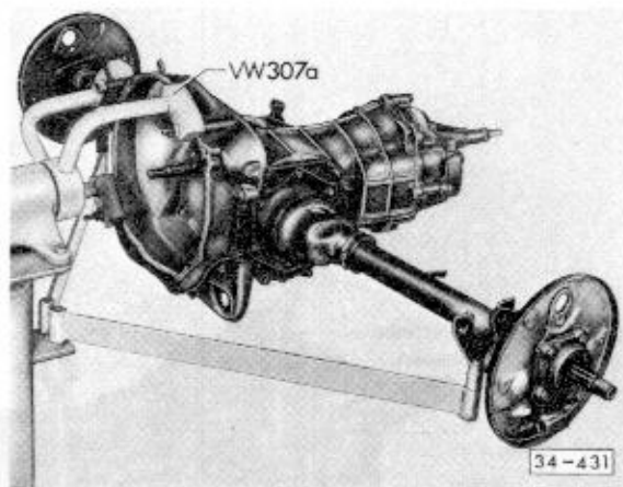
Abb. 1 Getriebe in den Montagebock spannen AUDI NSU: VW 540
