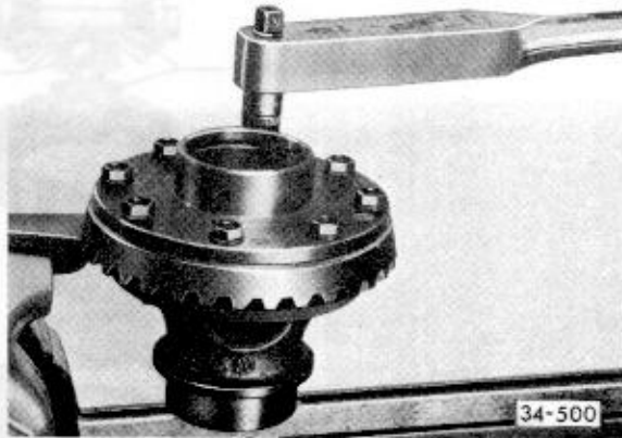
Abb. 4 Tellerradschrauben über Kreuz mit 60 Nm (6 mkg) anziehen
