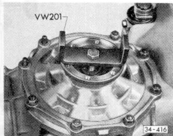
Abb. 13 Sicherungsring einsetzen
