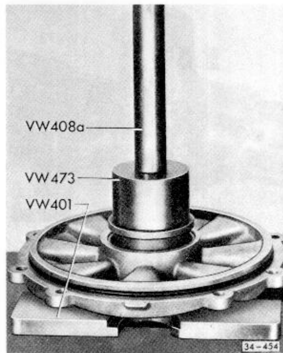
Abb. 5 Dichtring auspressen
