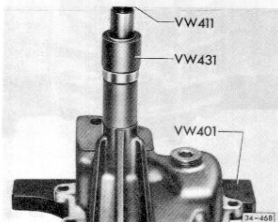
Abb. 2 Lagerbuchse mit Dichtring einpressen
