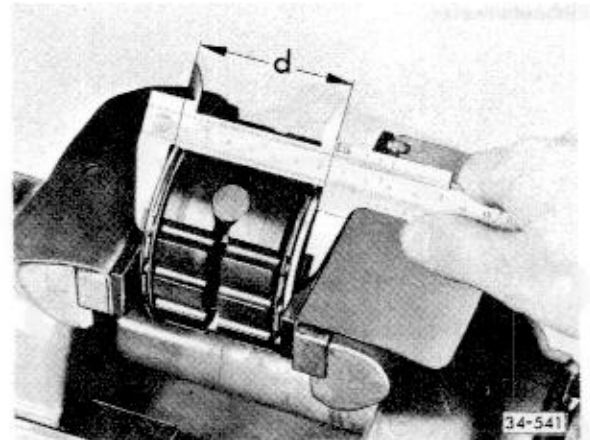
Abb. 7 Dicke des Lamellenpaketes – Maß d – ermitteln (mit 2 Außenlamellen 1,9 mm dick, jedoch ohne Tellerfedern)
