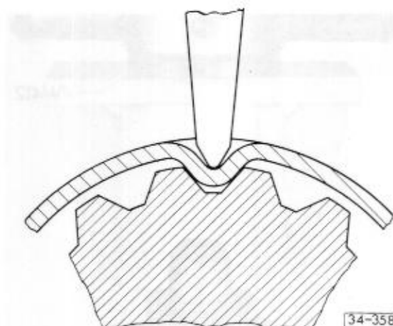
Abb. 7 Rundmutter sichern.
