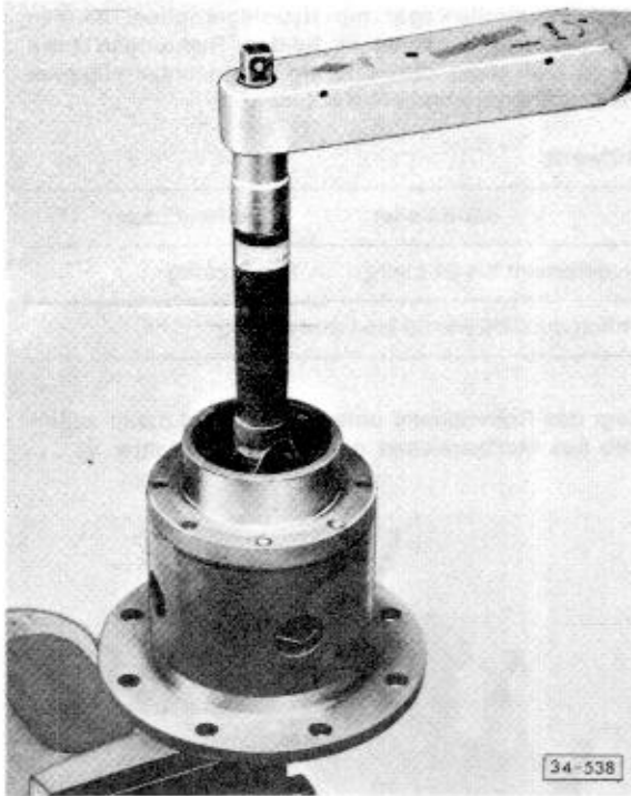
Abb. 9 Nach dem Zusammenbau Durchdrehmoment prüfen
