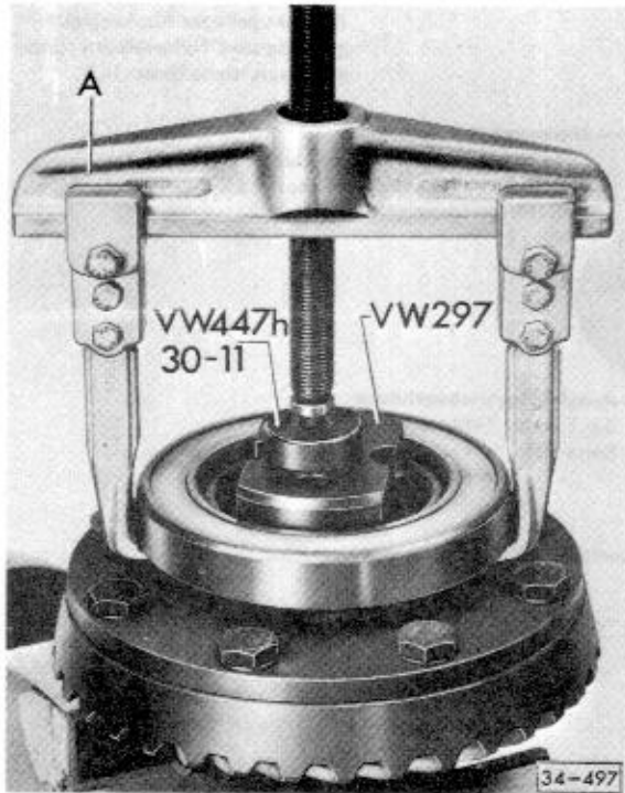
Abb. 1 Rillenkugellager abziehen
