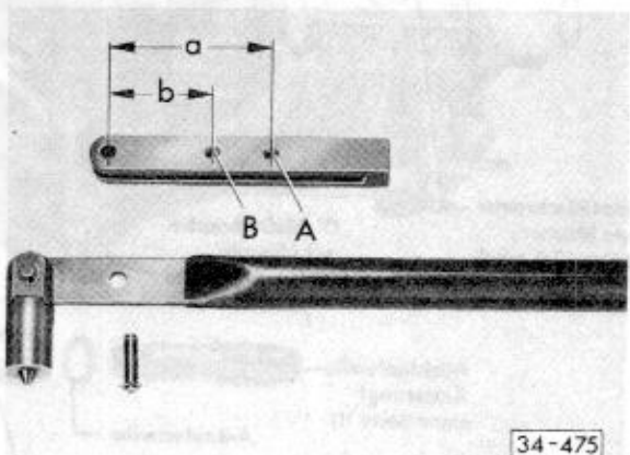
Abb. 6 Ausdrückhebel umarbeiten
