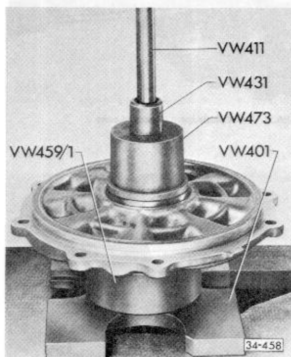
Abb. 9 Außenring/Kegelrollenlager für Ausgleichgetriebe einpressen
