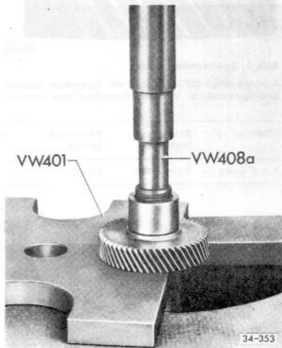
Abb. 2 Zahnrad für 4. Gang mit Innenlauftring/Nadel-lager abpressen
