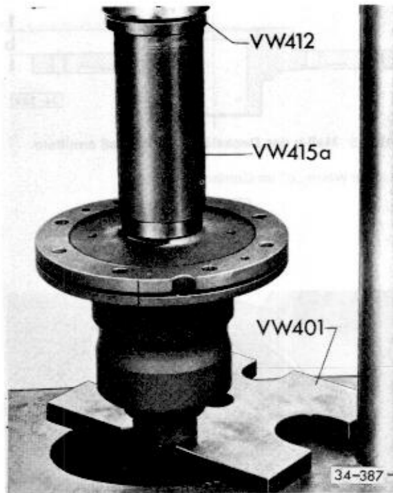
Abb. 3 Deckel aufpressen
