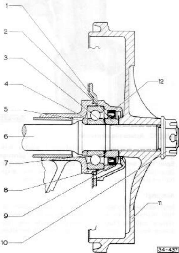
Abb. 7 Einbaulage der Radlagerung
