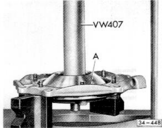
Abb. 3 Rillenkugellager für Ausgleichgetriebe auspressen
