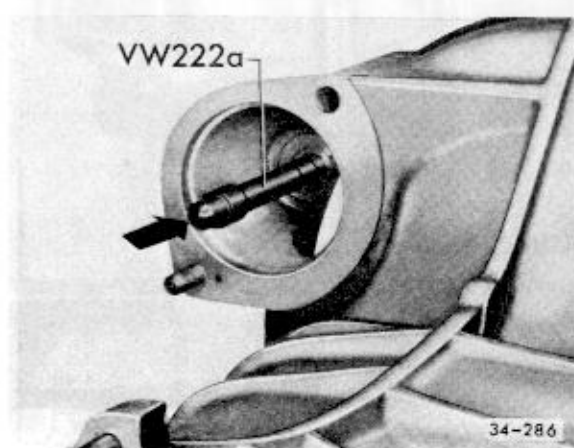
Abb. 9 Lagerbuchse für Anlasser bündig eintreiben
