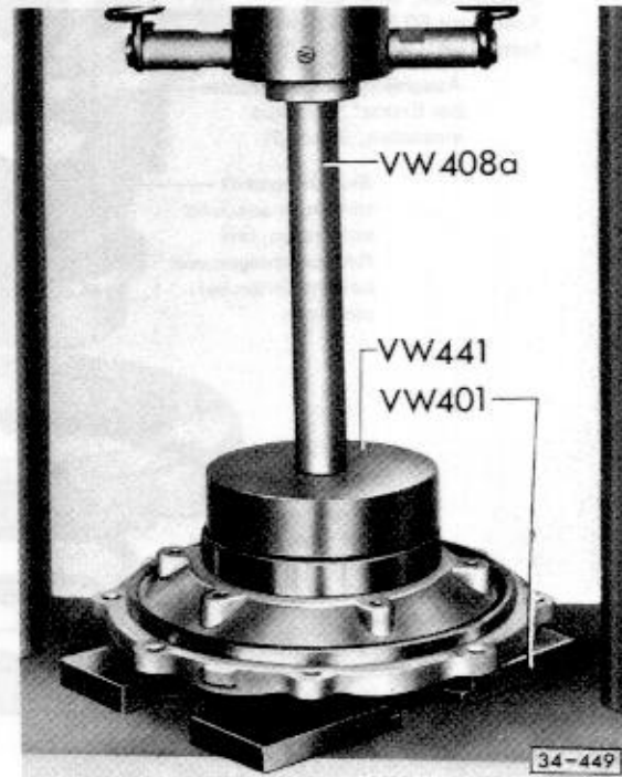
Abb. 4 Rillenkugellager für Ausgleichgetriebe einpressen
