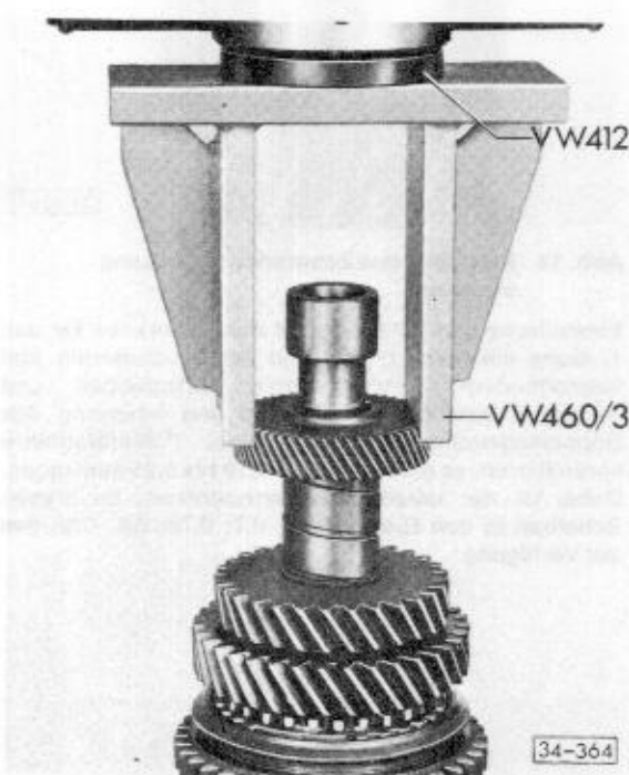
Abb. 14 Zahnrad für 4. Gang, Innenlauftring/ Nadellager und Sicherungsring einbauen
