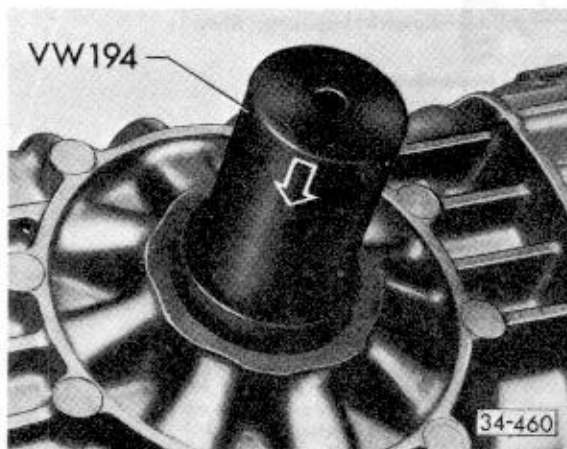
Abb. 11 Dichtring eintreiben
