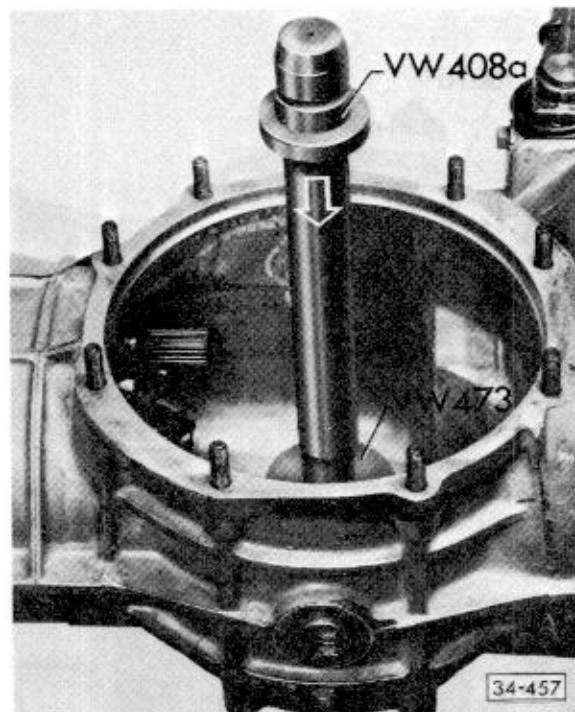
Abb. 8 Außenring/Kegelrollenlager für Ausgleichgetriebe mit Plastikhammer eintreiben
