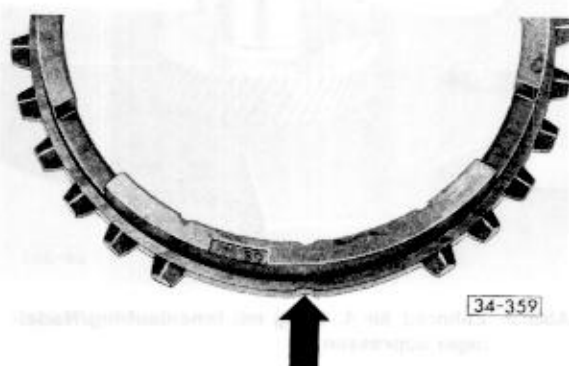
Abb. 9b 2. Gang: 3 Kerben (Pfeil).
