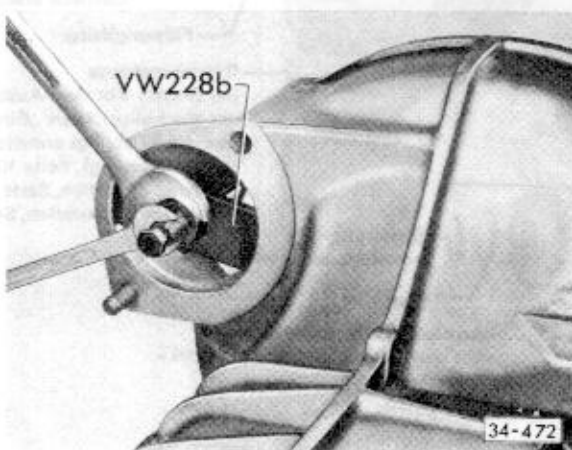
Abb. 3 Lagerbuchse für Anlasser ausziehen
