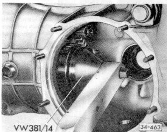
Abb. 2 Spannmutter ab- bzw. anschrauben Anschrauben: mit 220 Nm (22 mkg) anziehen, lösen und mit 220 Nm festziehen.
