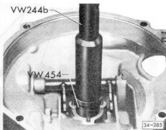
Abb. 10 Dichtring für Antriebswelle eintreiben
