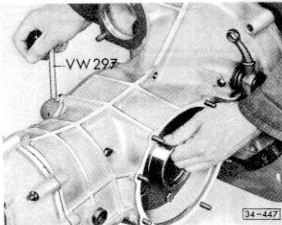
Abb. 2 Ausgleichgetriebe herausdrücken
