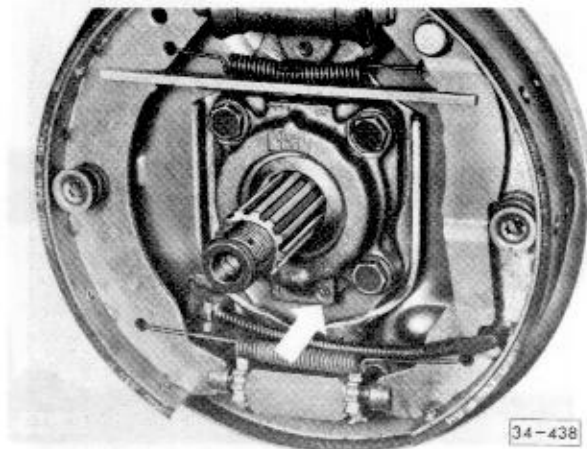
Abb. 8 Deckel für Hinterradlager so einbauen, daß die Öltropfnase (Pfeil) nach unten zeigt
